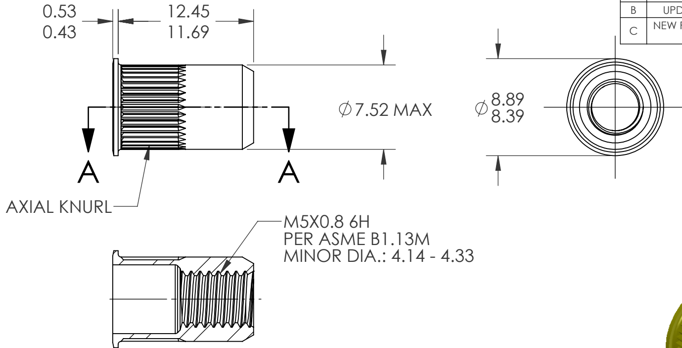
SECTION A-A SCALE 3 : 1
