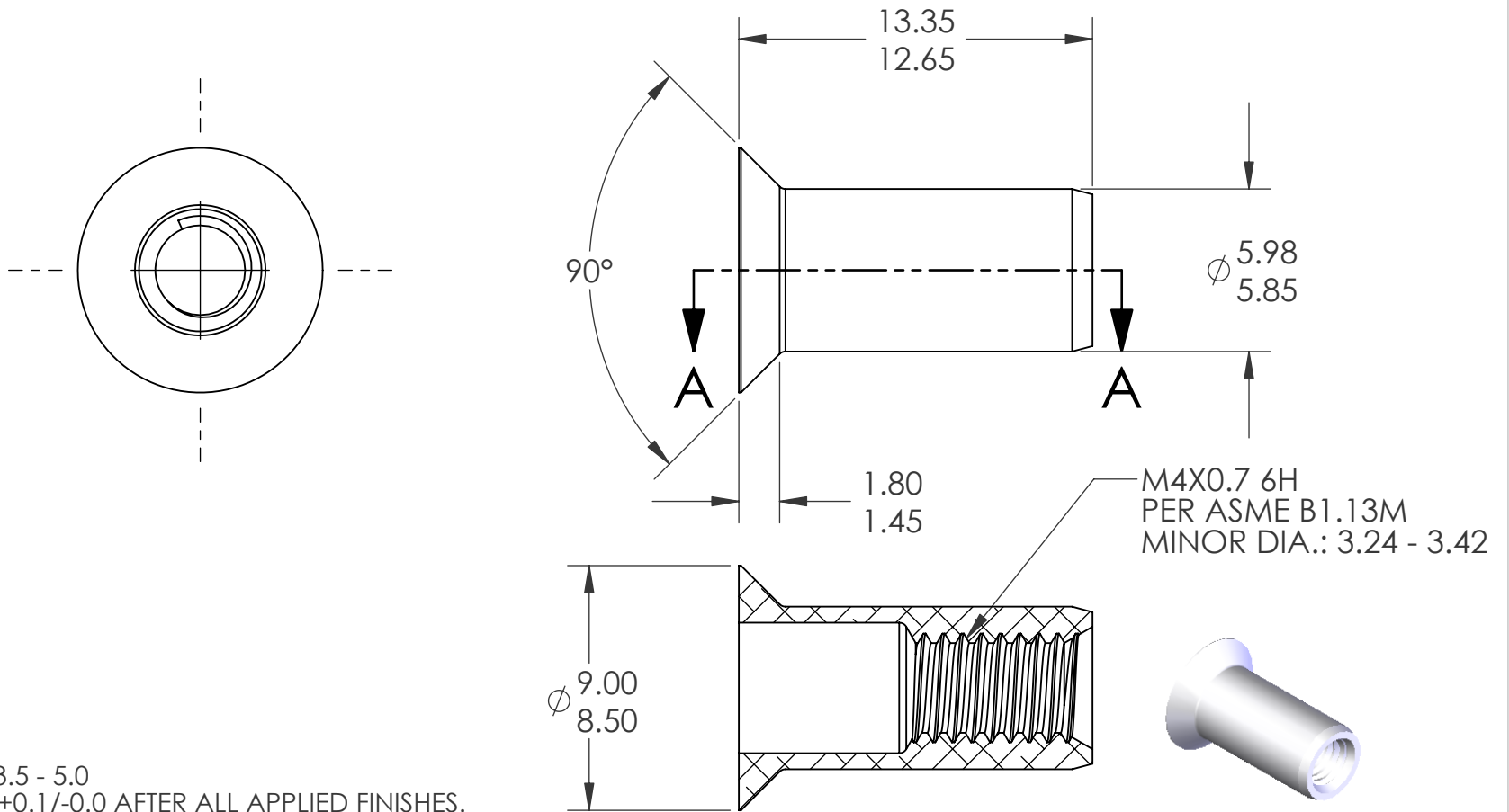
SECTION A-A
