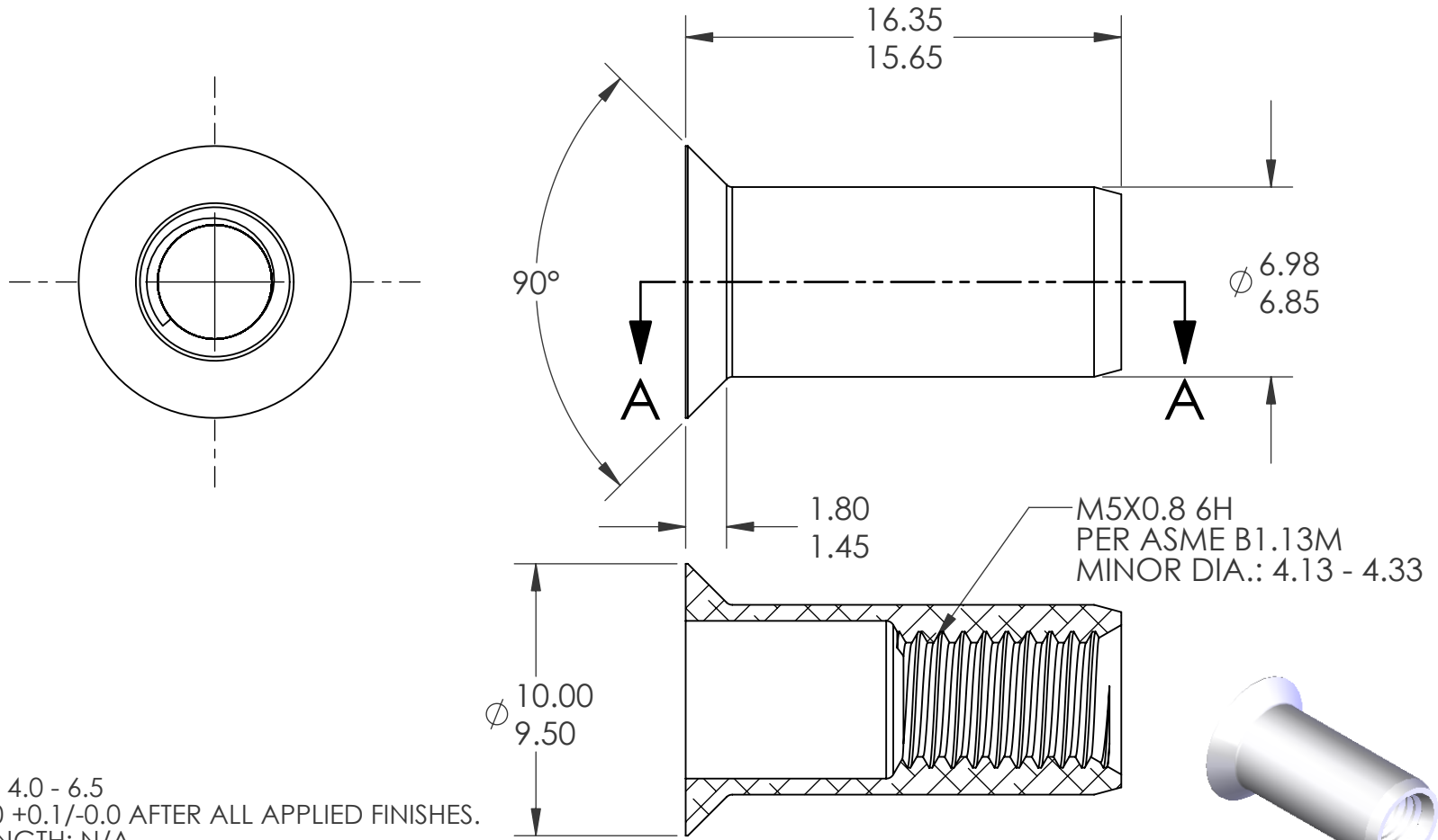
SECTION A-A
