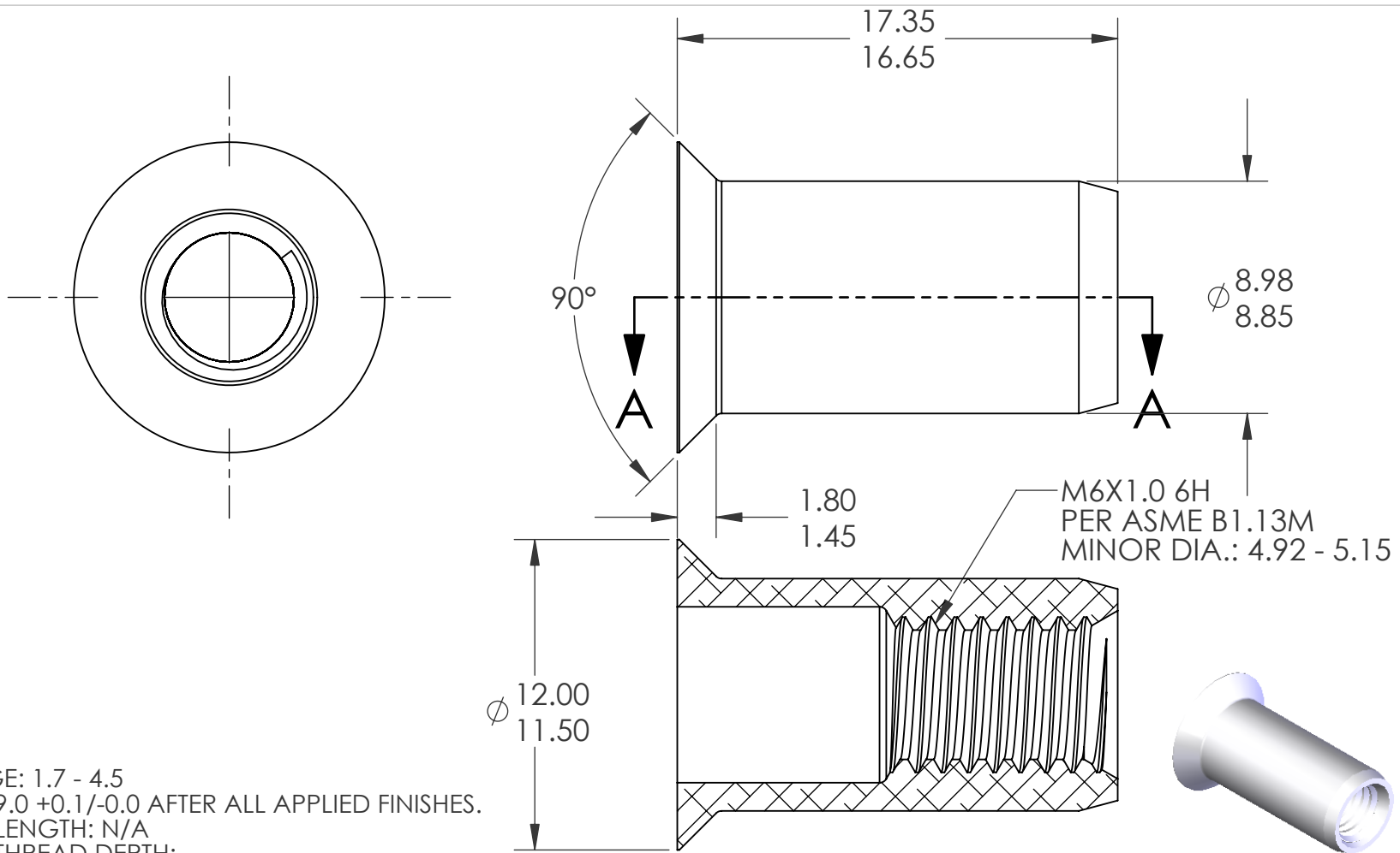
SECTION A-A
