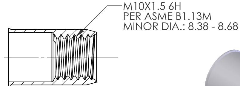
SECTION A-A SCALE 2 : 1
