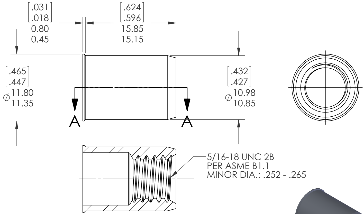
SECTION A-A SCALE 3 : 1
