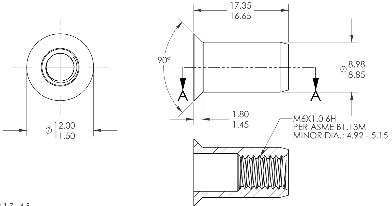
SECTION A-A
